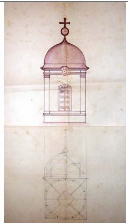
Toronymsiak ácsmunka terv – 1853 – Takáts István és József átsmesterek
